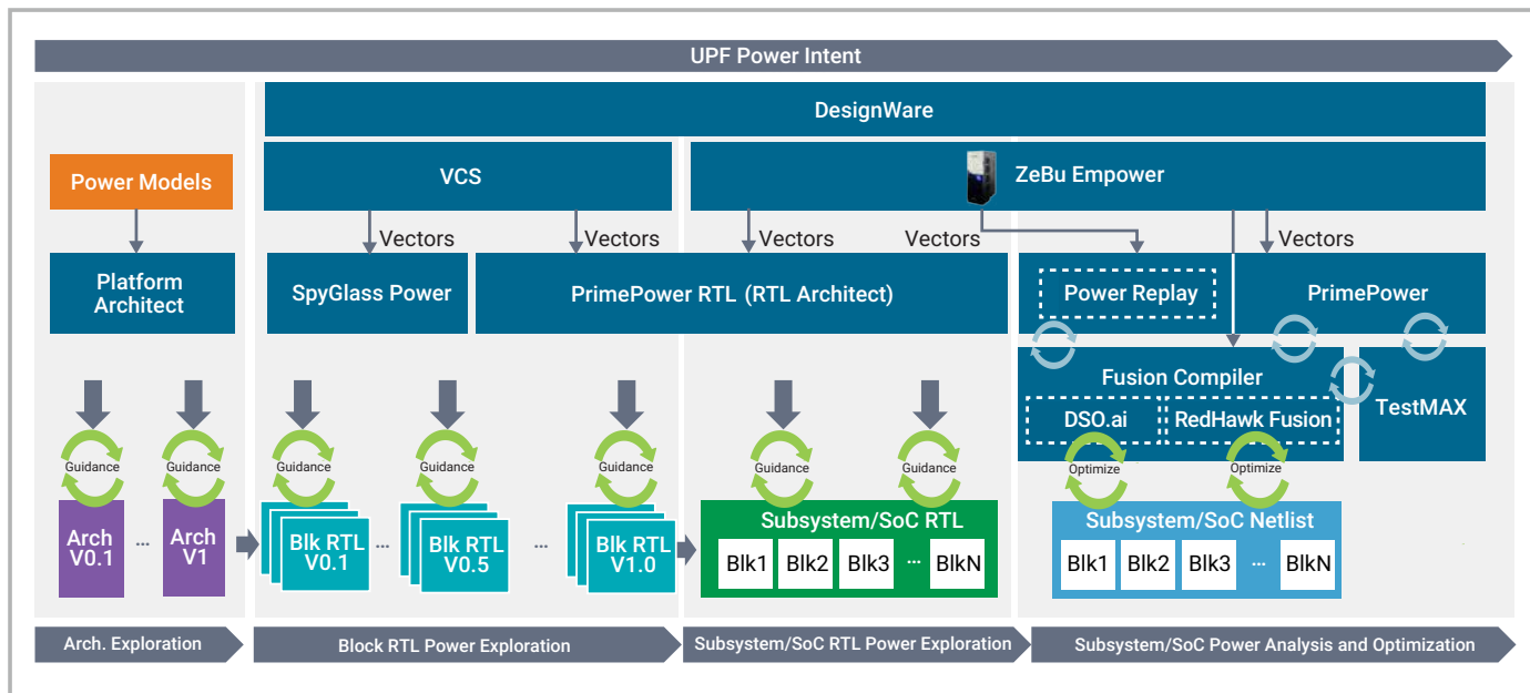
圖5：以軟體驅動的功耗探索、分析及優化
