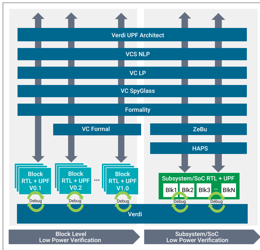
圖6：新思科技低功耗驗證
