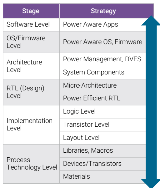
圖2：端到端節能設計流程
