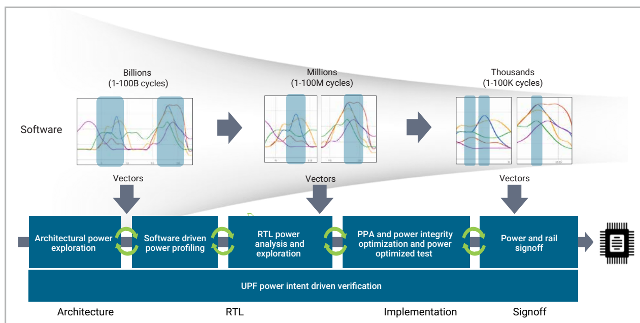
圖3：低功耗設計流程
