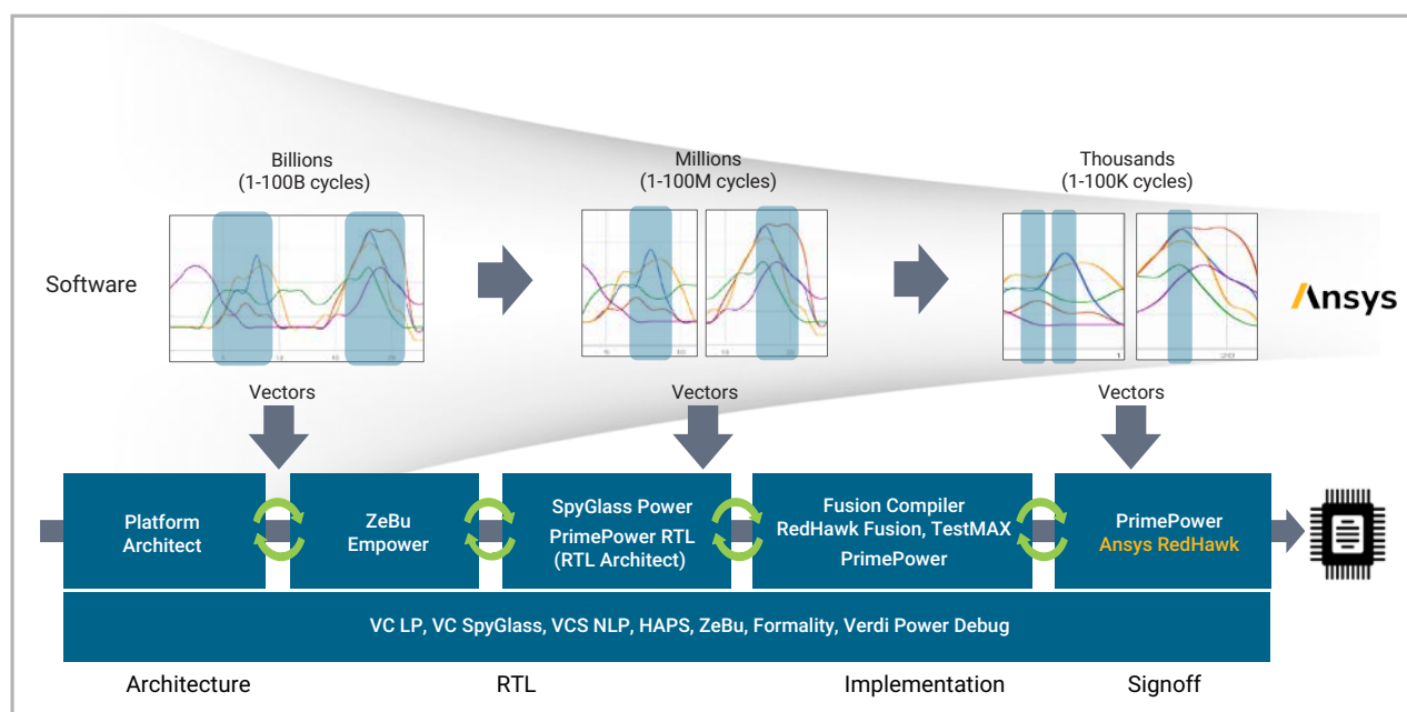
圖4：新思科技低功耗解決方案
